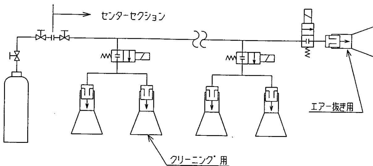
図4 配管の概念図
