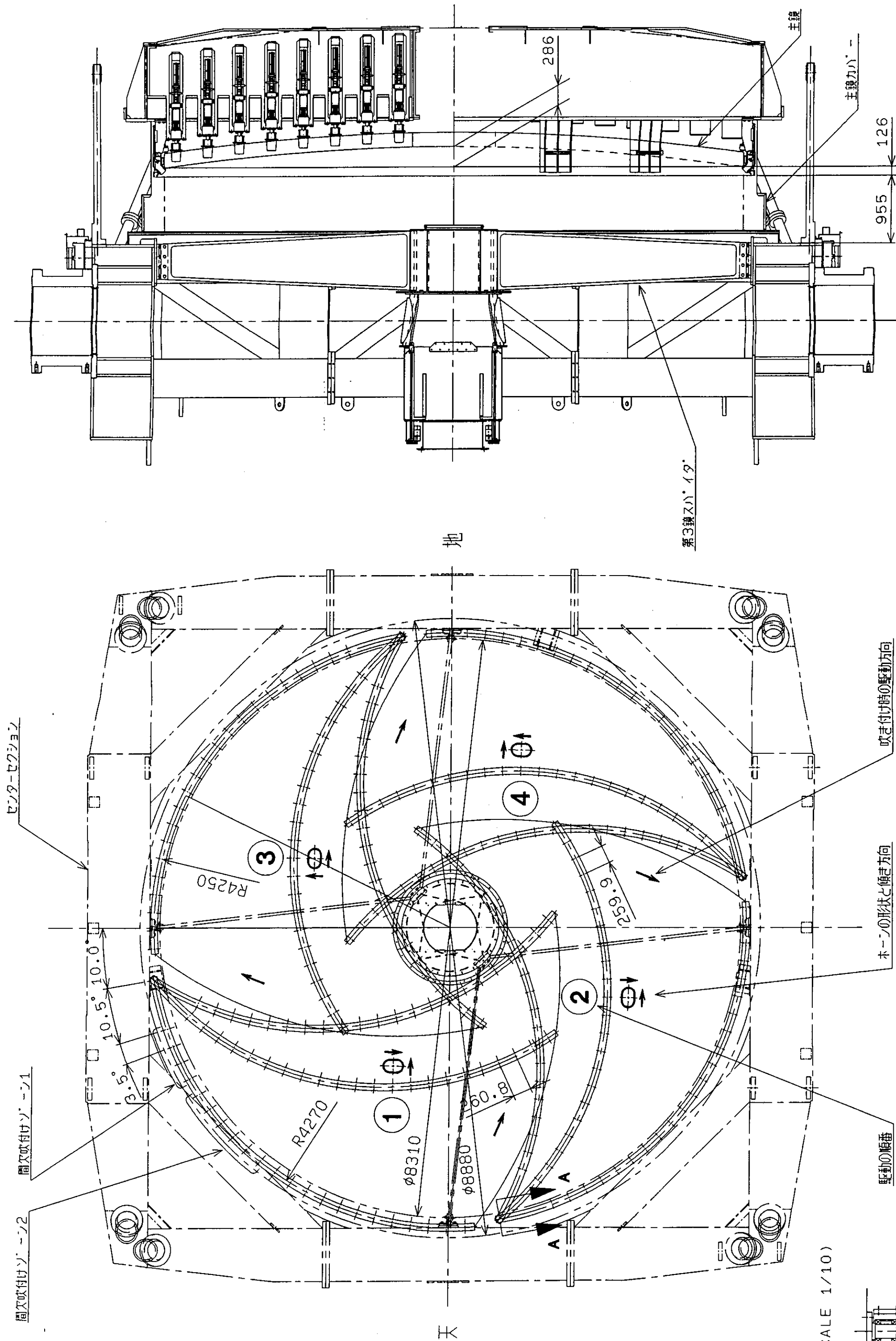
図1 主鏡クリーニング装置 概念図(1/3) (SCALE 1/50)
