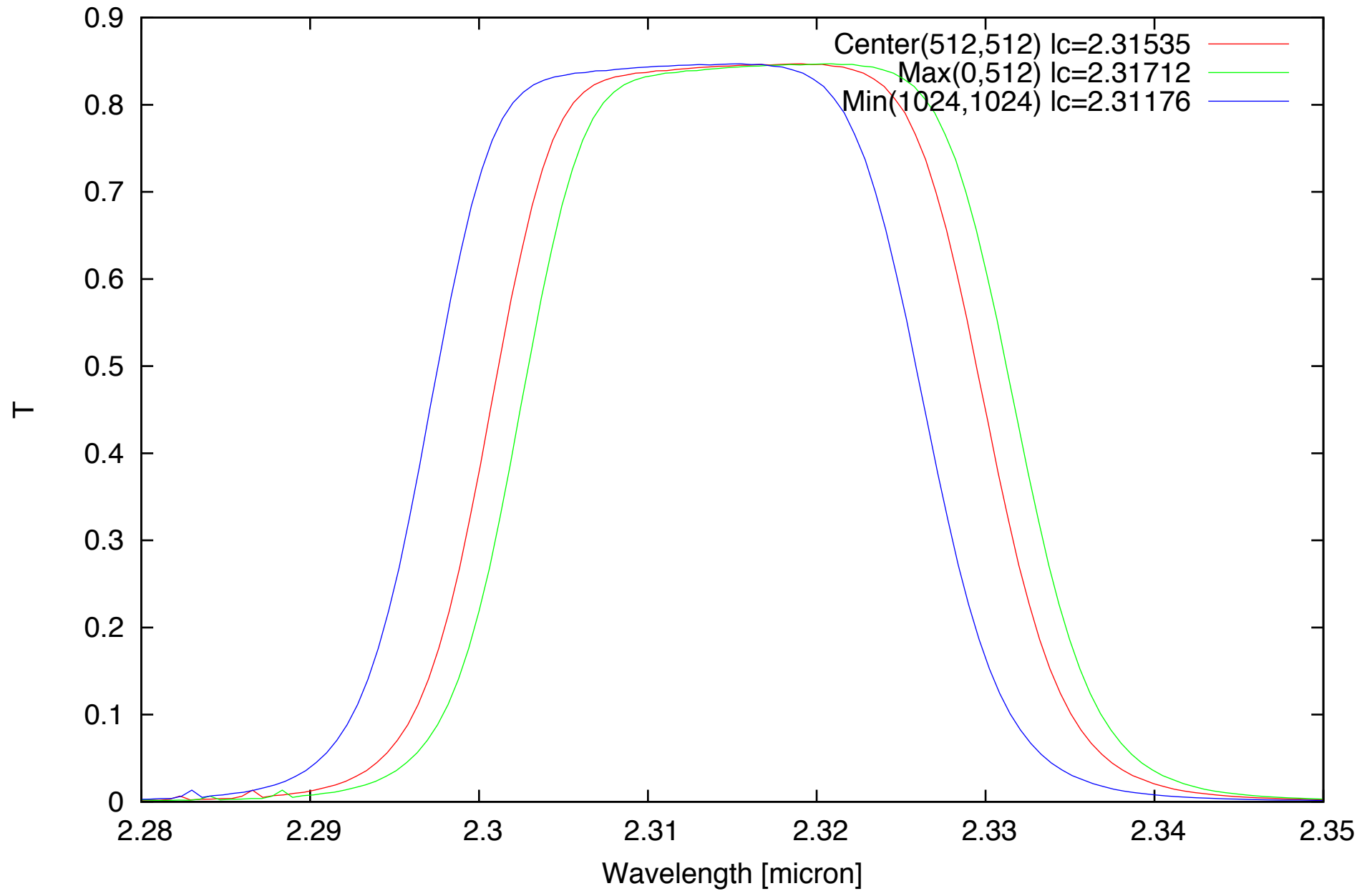
IRCS NB231 filter Width=298A
